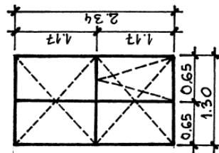
PARAPET WEWNĘTRZNY Z KONGLOMERATU MARMUROWEGO SZEROKOŚĆ 0,30 m. SZT. 6
